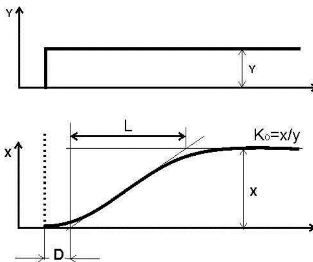
Рисунок 10.1 - Переходная функция объекта регулирования с самовыравниванием
