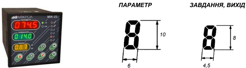
Рисунок А.1 – Внешний вид микропроцессорного регулятора.
