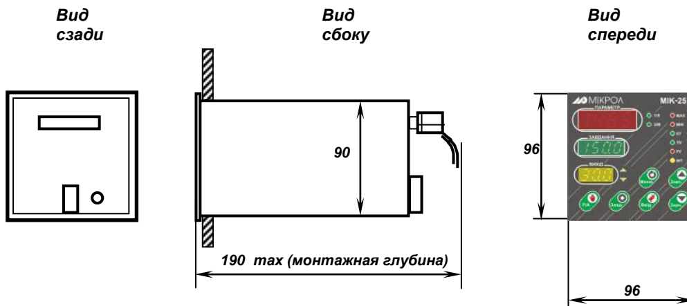
Рисунок А.1 – Внешний вид микропроцессорного регулятора.
