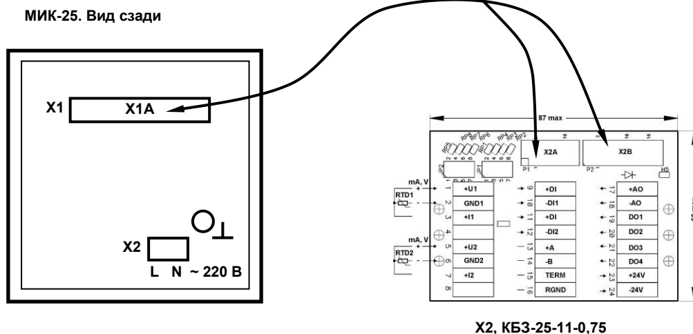
Рисунок Б.1 - Подключение клеммно-блочного соединителя КБ3-25-11-0,75 к регулятору МИК-25
