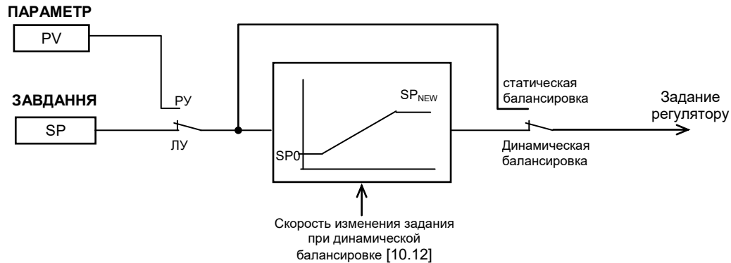
Рисунок 6.4.3 – Функциональная схема балансировок регулятора МИК-25
