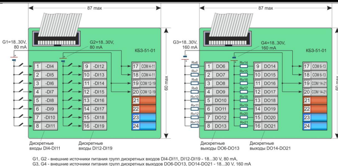
Рисунок 8.4.18 - Подключение сигналов модуля расширения МР-52-32 с помощью клеммно-блочных соединителей КБ3-51-01 (транзисторные выходы)
