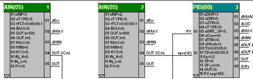
Рисунок 2.6 – Связные параметры
