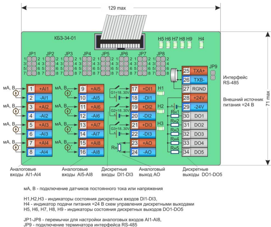
Рисунок 8.2.2 - Подключение клеммно-блочного соединителя КБЗ-34-01 к контроллеру МИК-52
