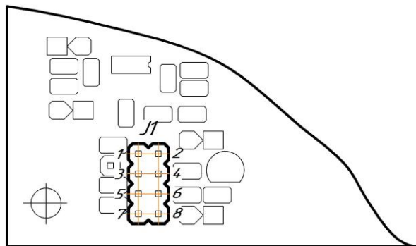
Рисунок 8.3.1 – Положение переключателей на плате контроллера МИК-52
