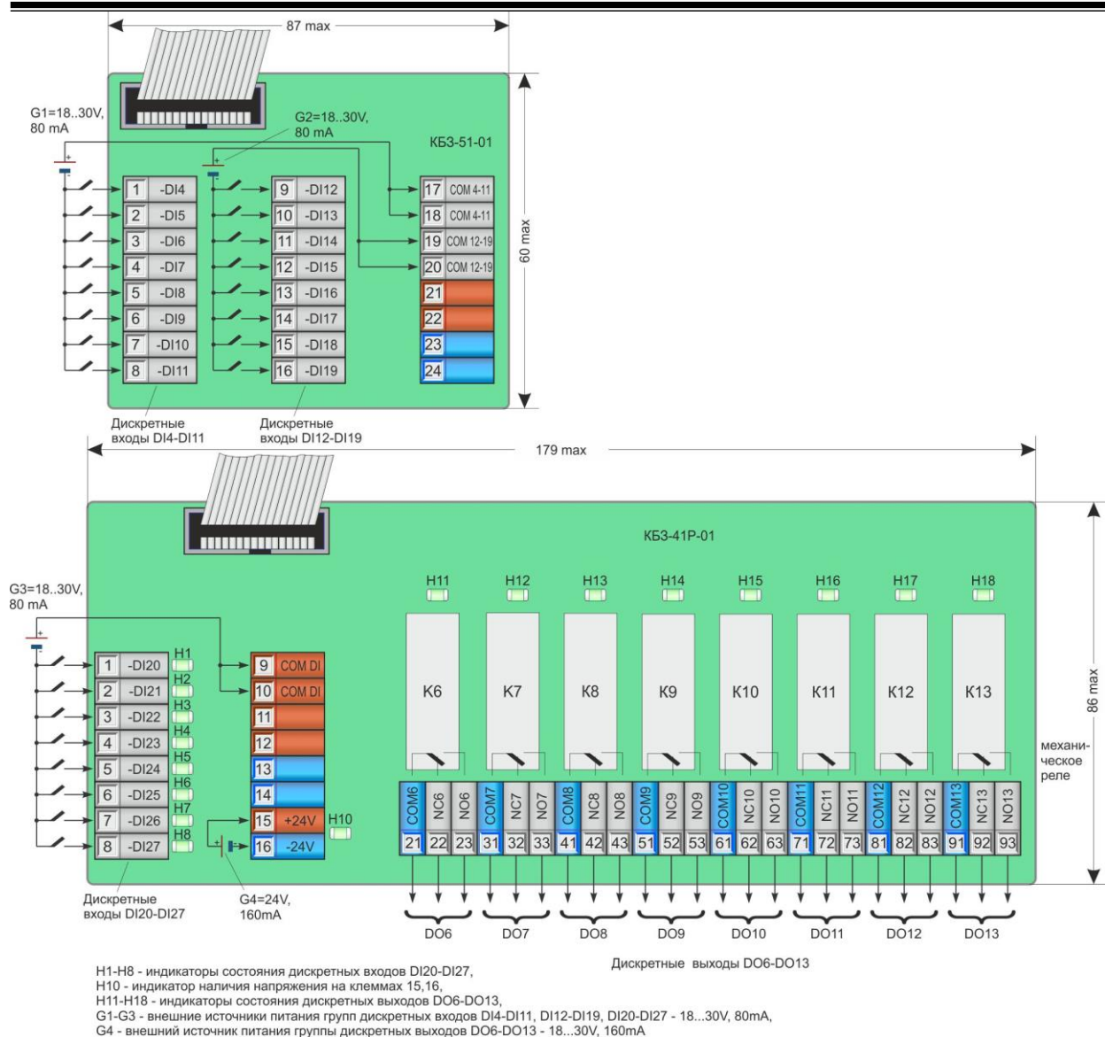
Рисунок 8.4.17 - Подключение сигналов модуля расширения МР-52-31 с помощью клеммно-блочного соединителя KB3-41P-01 (KB3-51-01+KB3-40P-01)
