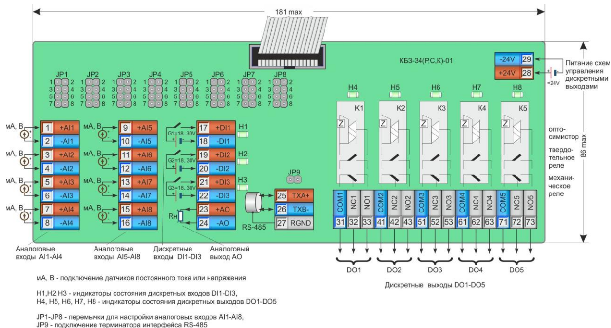
Рисунок 8.2.1 - Подключение клеммно-блочного соединителя КБЗ-34(Р,С,К)-01 к контроллеру МИК-52
