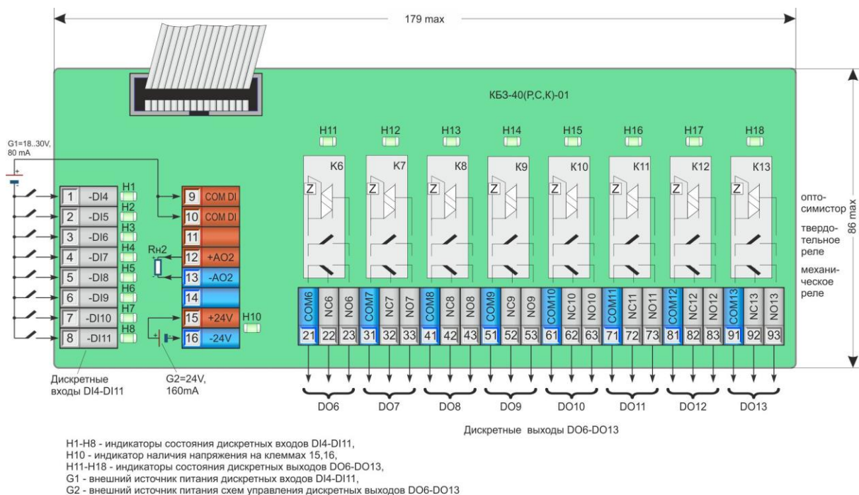
Рисунок 8.4.12 - Подключение сигналов модуля расширения МР-52-13 (МР-51-13) с помощью клеммно-блочного соединителя КБ3-40(Р,С,К)-01
