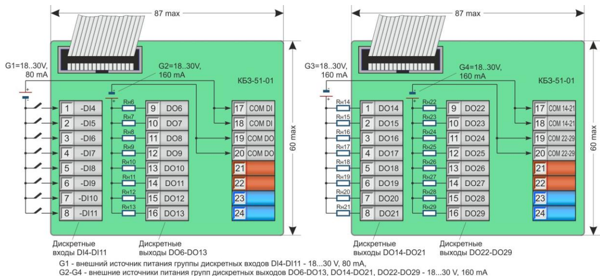
Рисунок 8.4.20 - Подключение сигналов модуля расширения МР-52-33 с помощью клеммно-блочных соединителей KB3-51-01 (транзисторные выходы)
