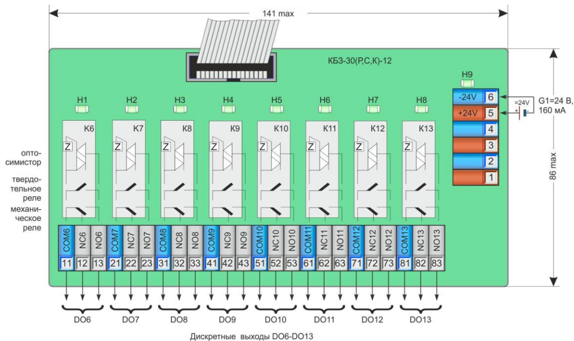
Рисунок 8.4.3 - Подключение сигналов модуля расширения МР-52-03 (МР-51-03) с помощью клеммно-блочного соединителя КБЗ-30(Р,С,К)-12
