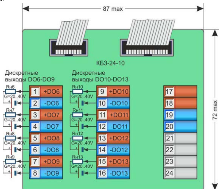
Рисунок 8.4.2 - Подключение сигналов модуля расширения МР-52-03 (МР-51-03) с помощью клеммно-блочного соединителя КБЗ-24-10
