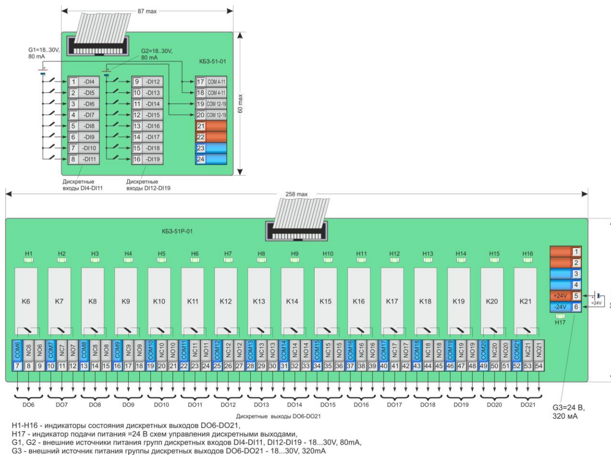
Рисунок 8.4.19 - Подключение сигналов модуля расширения МР-52-32 с помощью клеммно-блочного соединителя КБ3-51P-01 (КБ3-51-01+КБ3-54P-01)
