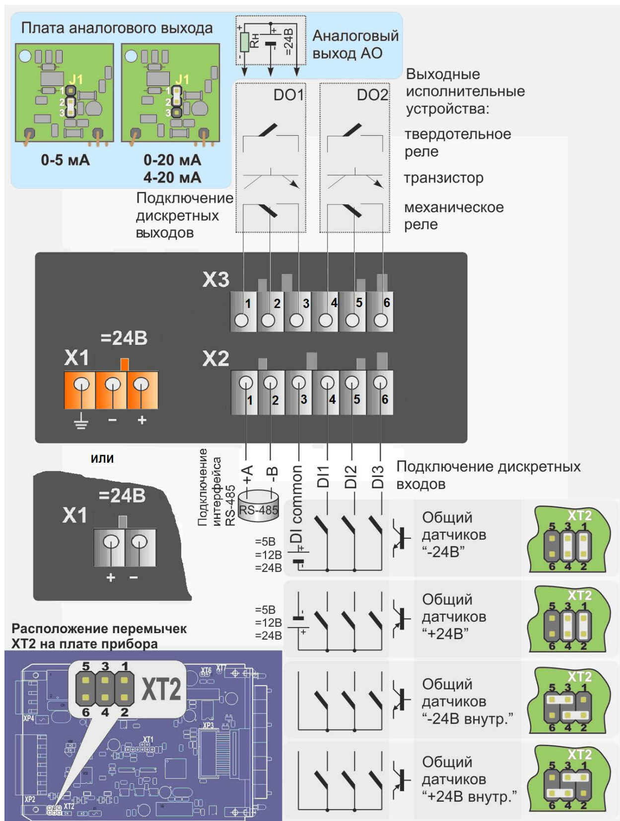
Рисунок Б.1.2 - Подключение внешних цепей счетчика МТЛ-32. Вид сзади. Исполнение на напряжение 24 В постоянного тока(такое же самое исполнение для счетчиков на 36 В постоянного тока)
