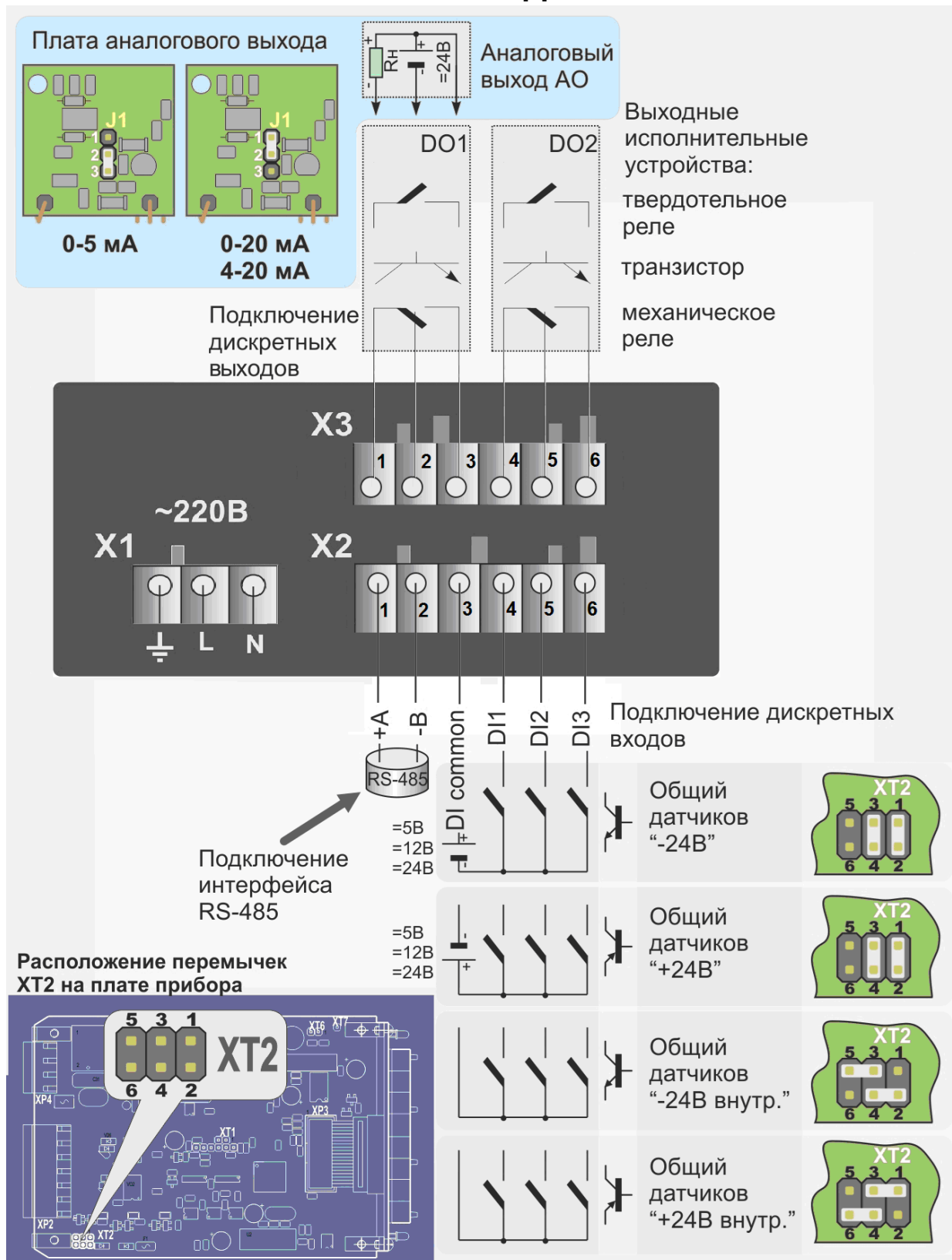
Рисунок Б.1.1 - Подключение внешних цепей счетчика МТЛ-32. Вид сзади. Исполнение на напряжении 220 В переменного тока
