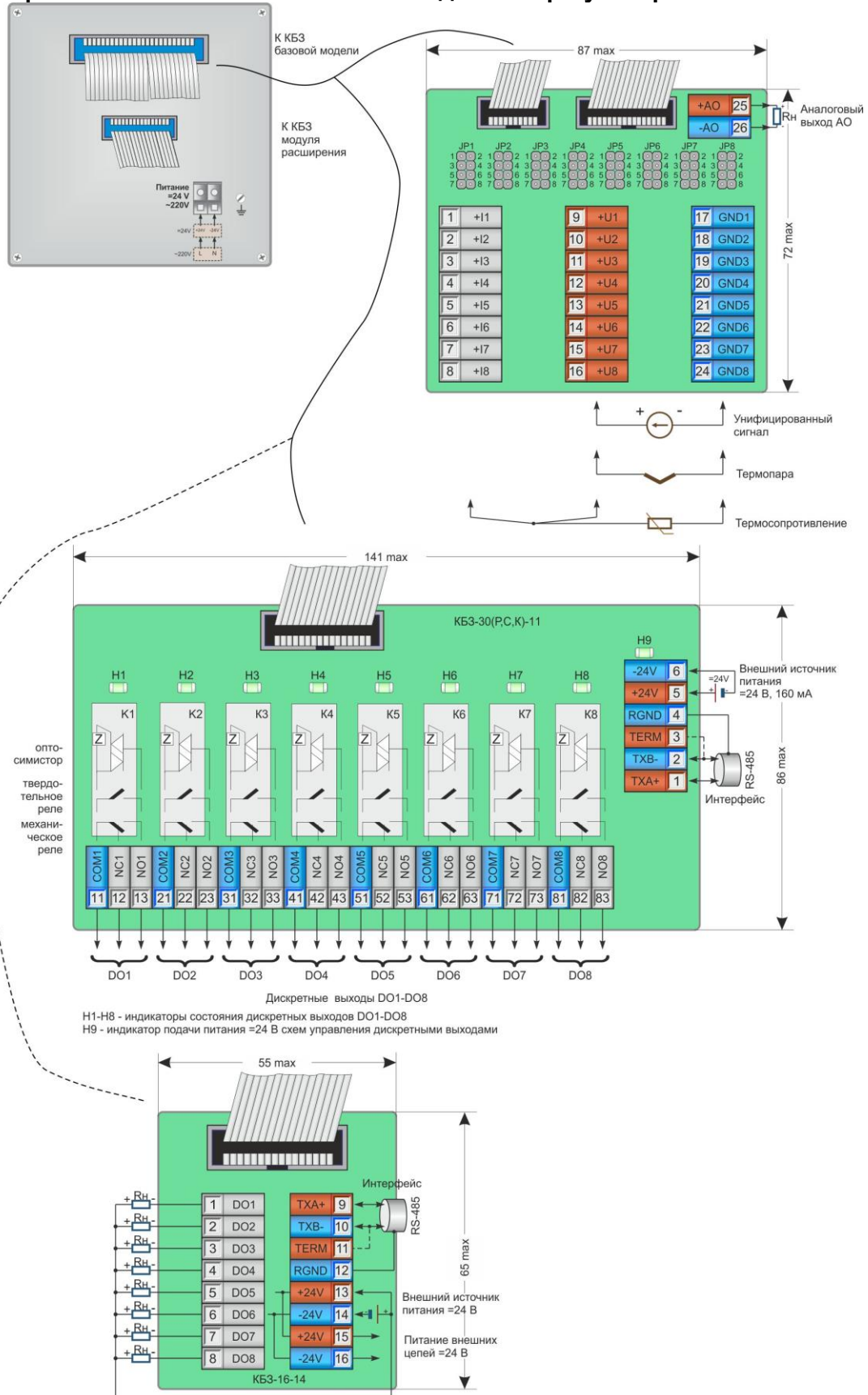
Рисунок Б.1 - Подключение клеммно-блочных соединителей КБЗ-24-17, КБЗ-30P(C,K)-11, КБЗ-16-14 к регулятору МТР-8
