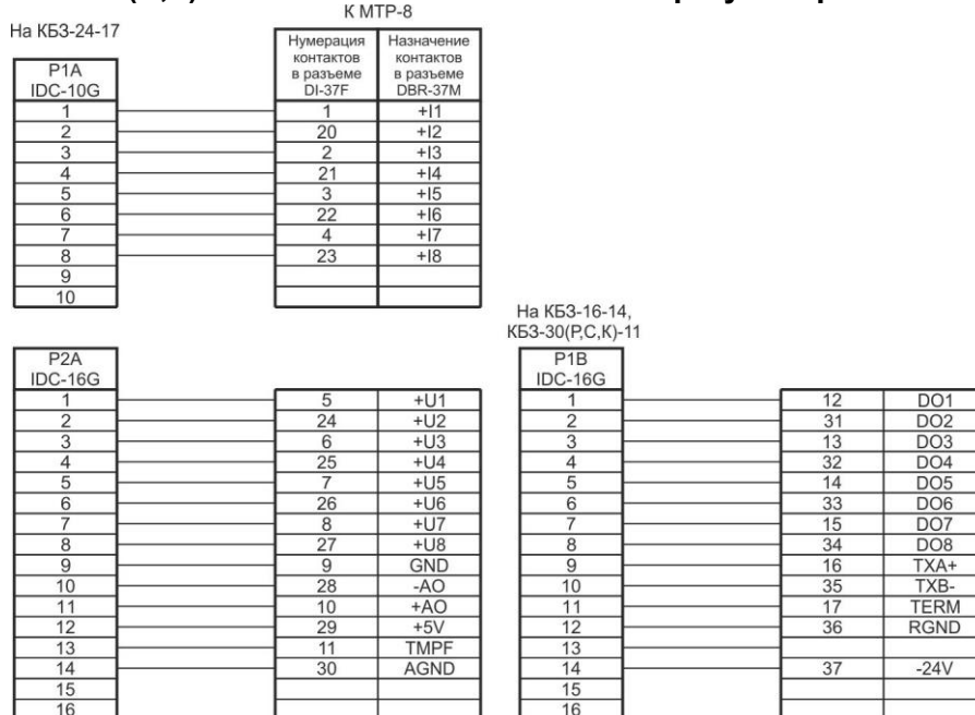
Рисунок Б.2 - Схема распыки кабеля клеммно-блочных соединителей КБЗ-24-17, КБЗ-30(Р,С,К)-11, КБЗ-16-14
