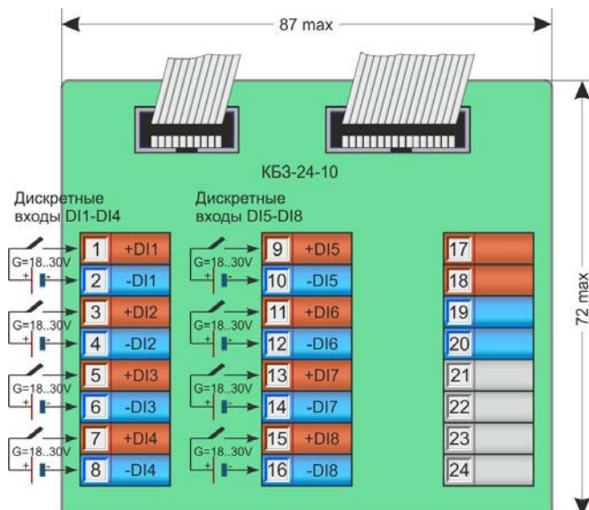
Рисунок Б.4.1 - Подключение сигналов модуля расширения МР-51-01 с помощью клеммно-блочного соединителя KB3-24-10
