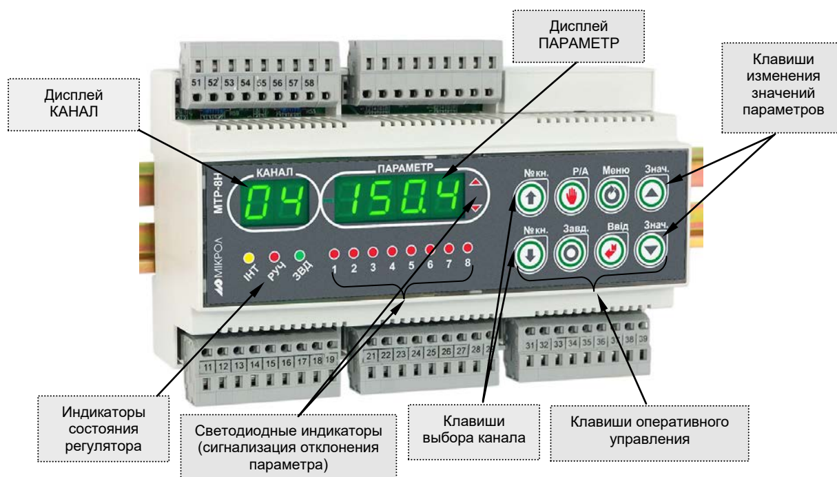
Рисунок 3.1 - Внешний вид регулятора MTP-8H
