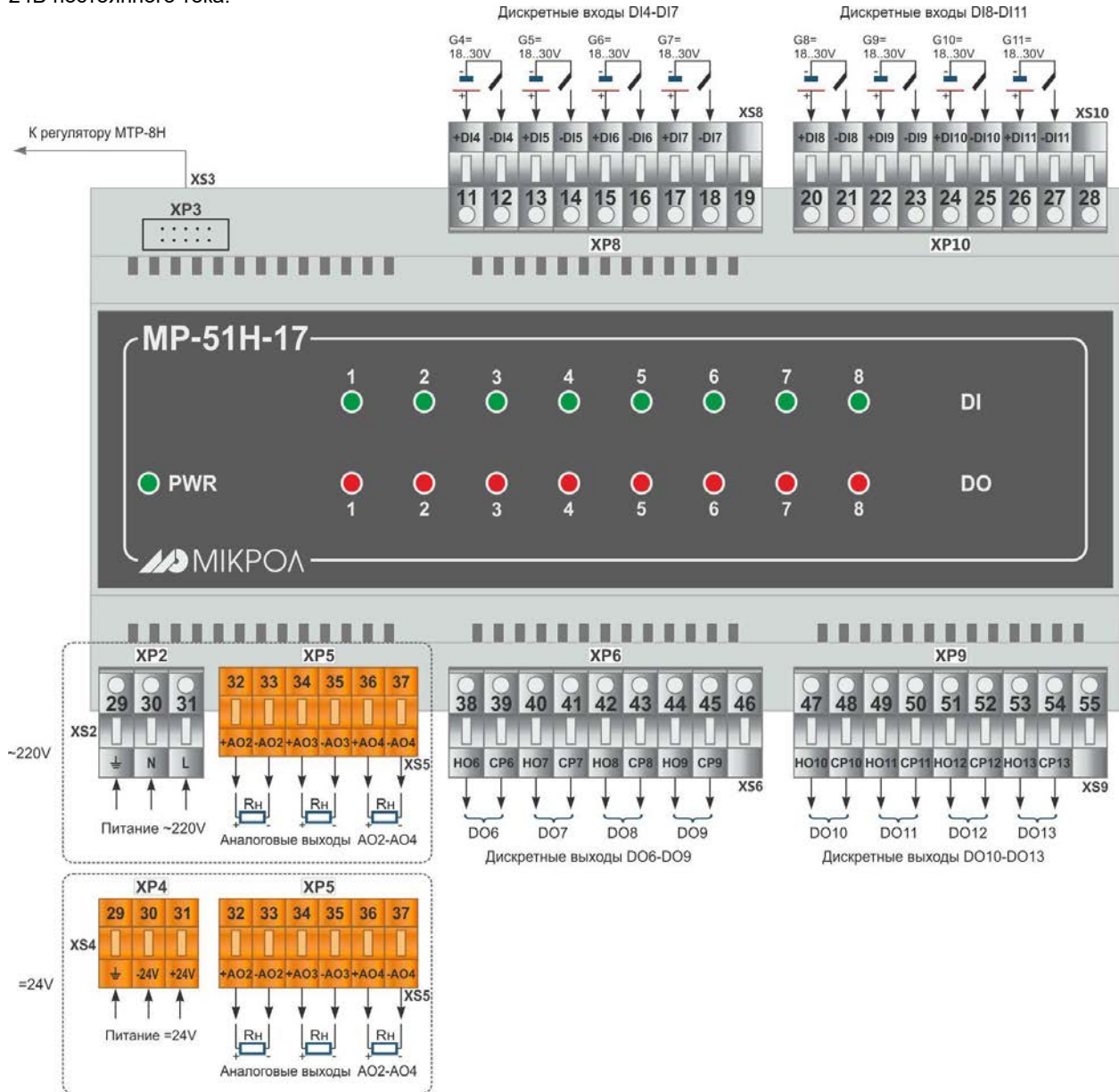
Рисунок Б.10 - Схема внешних соединений модуля расширения МР-51Н-17
