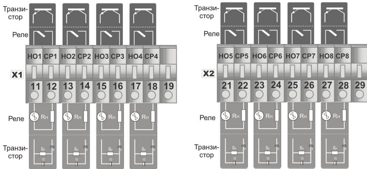
Рисунок Б.2 - Подключение дискретных нагрузок к регулятору МТР-8Н
