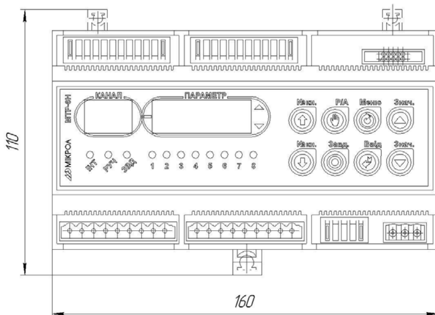
Рисунок А.1 - Габаритные и присоединительные размеры
