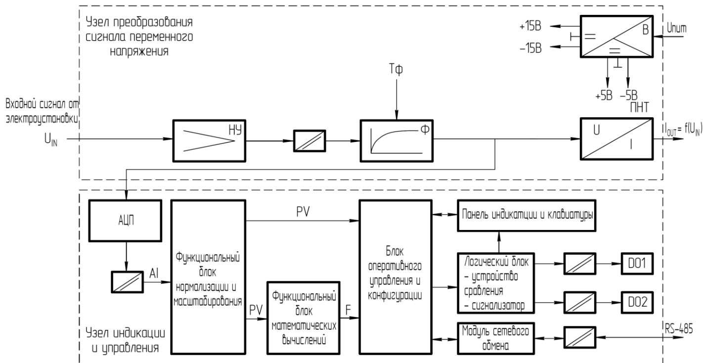
Рисунок 3.5.1 – Структурная схема преобразователя ПНС-12
