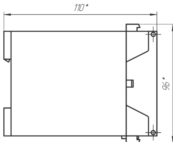
Рисунок А.1 – Внешний вид передней панели преобразователя ПНС-12
