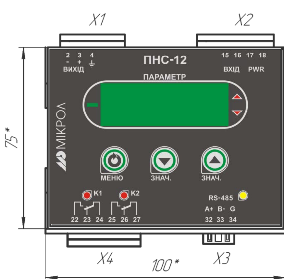
Рисунок А.1 – Внешний вид передней панели преобразователя ПНС-12
