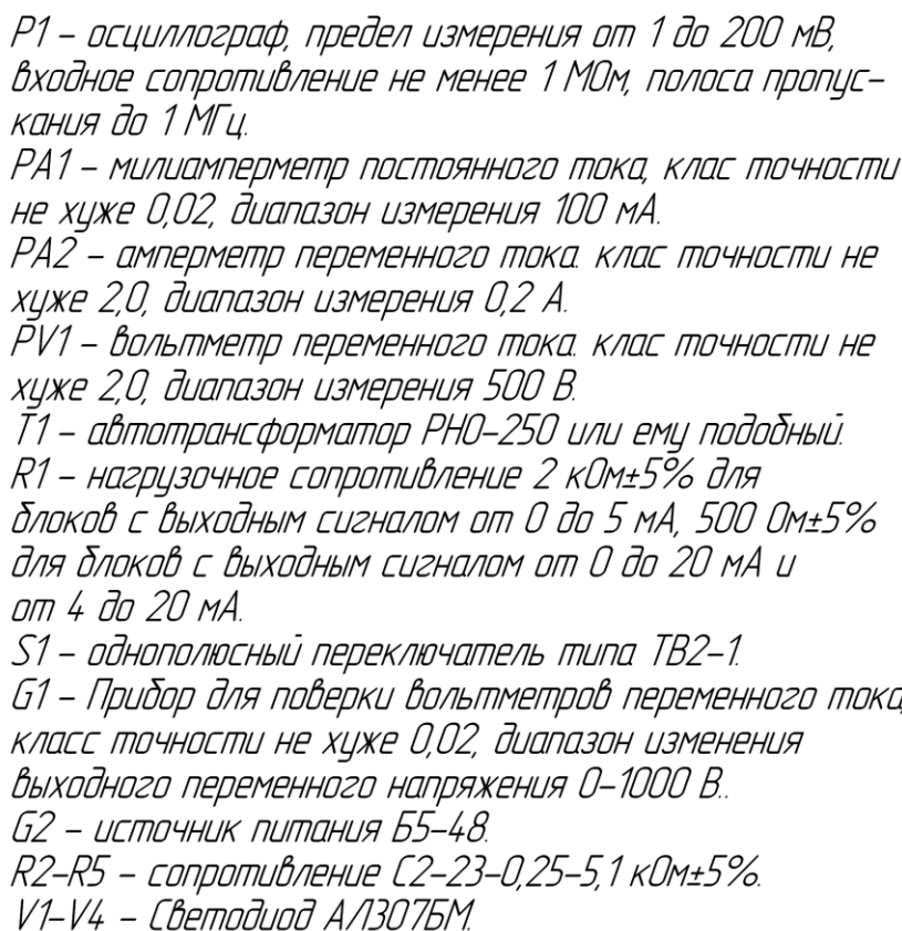
Рисунок Б.5 – Схема подключения преобразователя для проведения наладки
