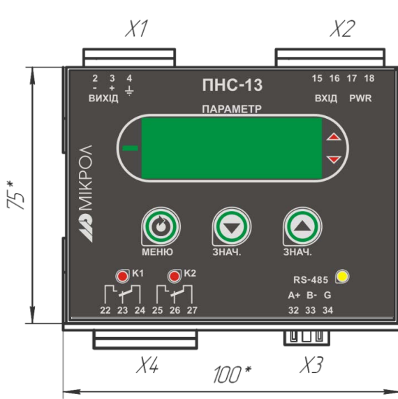
Рисунок А.1 – Внешний вид передней панели преобразователя ПНС-13
