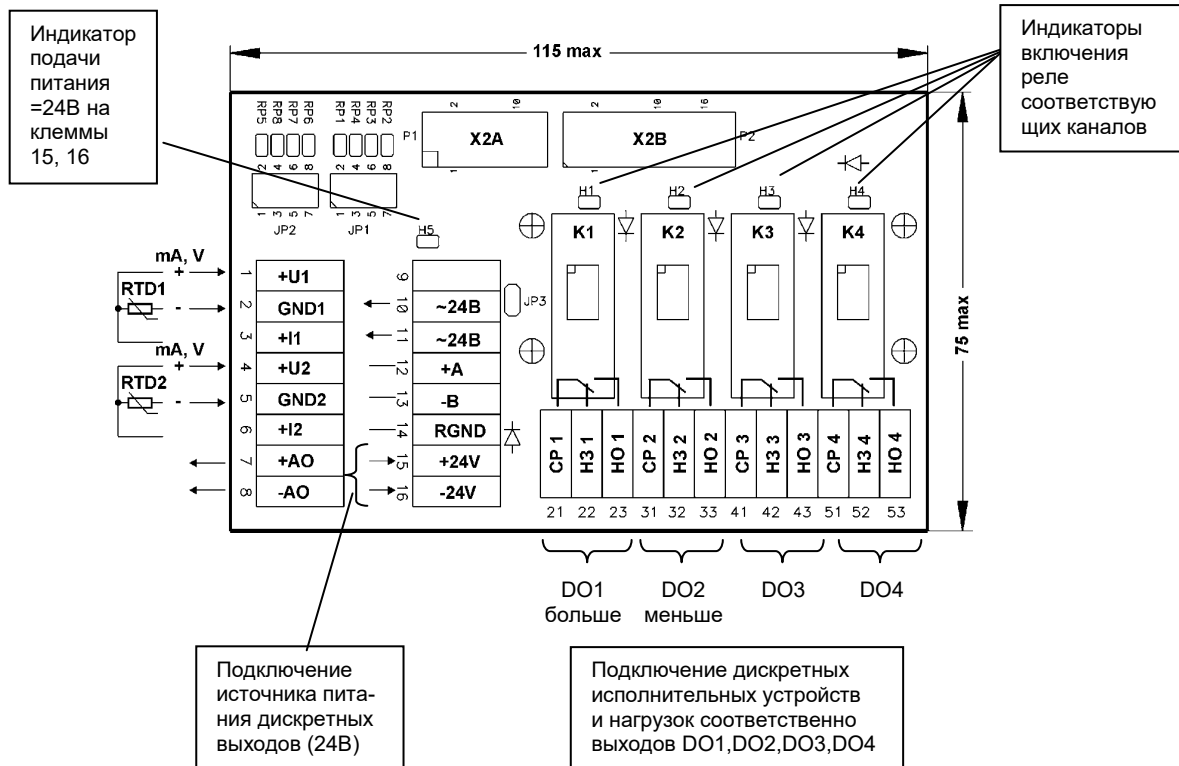
Рисунок Б.16 - Подключение дискретных нагрузок с помощью КБЗ-28Р-11
