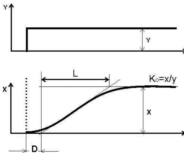
Рисунок 10.1 - Переходная функция объекта регулирования с самовывравниванием
