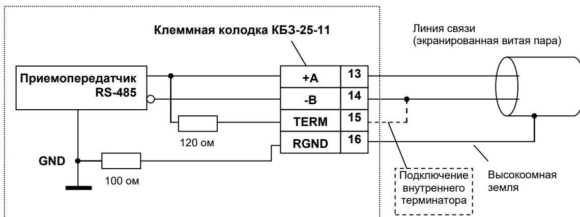
Рисунок Б.21 - Рекомендуемая схема подключения интерфейса RS-485 с помощью КБ3-25-11
