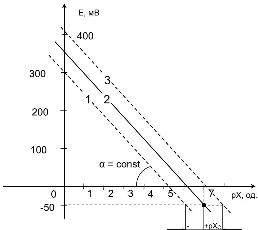
Рисунок 5.5. Коррекция смещения pX_{CM} электродной характеристики.
