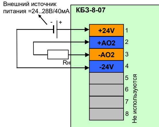
Рисунок Б.14 - Подключение сигналов модуля расширения МР-51-05 с помощью клеммно-блочного соединителя КБЗ-8-07
