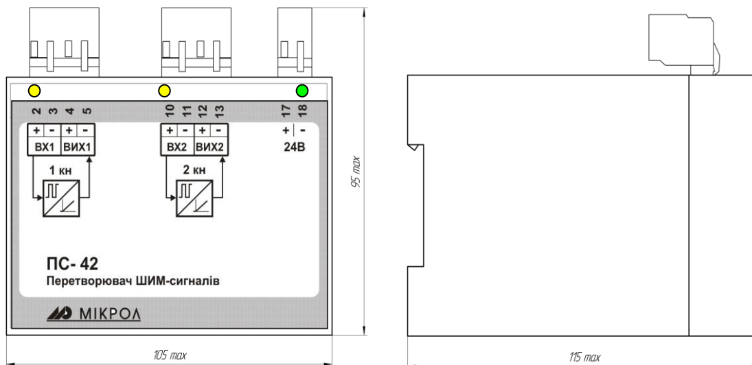
Рисунок 2.1 - Внешний вид и габаритные размеры ПС-42
