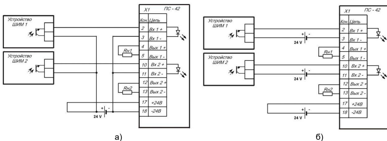
Рисунок 2.2 - Схема подключения блока ПС-42:
