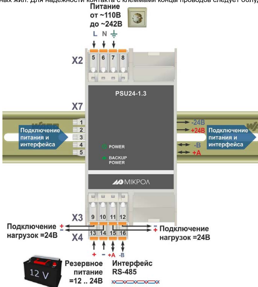
Рисунок 4.3 – Схема внешних соединений PSU24-1.3
