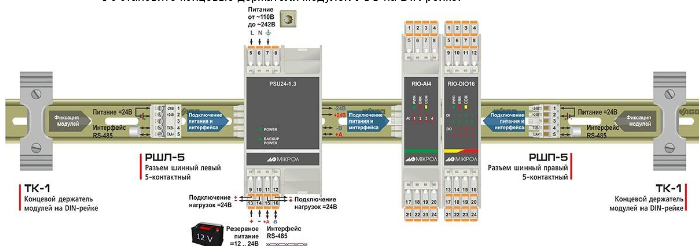
Рисунок 4.2 – Схема соединения блока питания с модулями УСО
