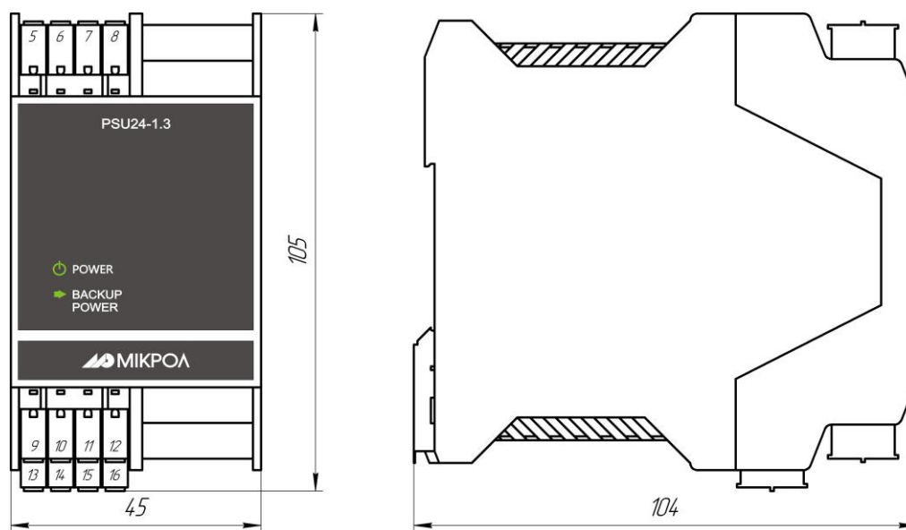
Рисунок 1.1 – Внешний вид и габаритные размеры PSU24-1.3
