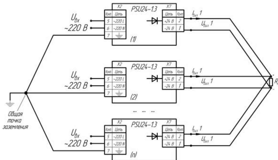
Рисунок 2.1 - Параллельное соединение блоков питания PSU24-1.3
