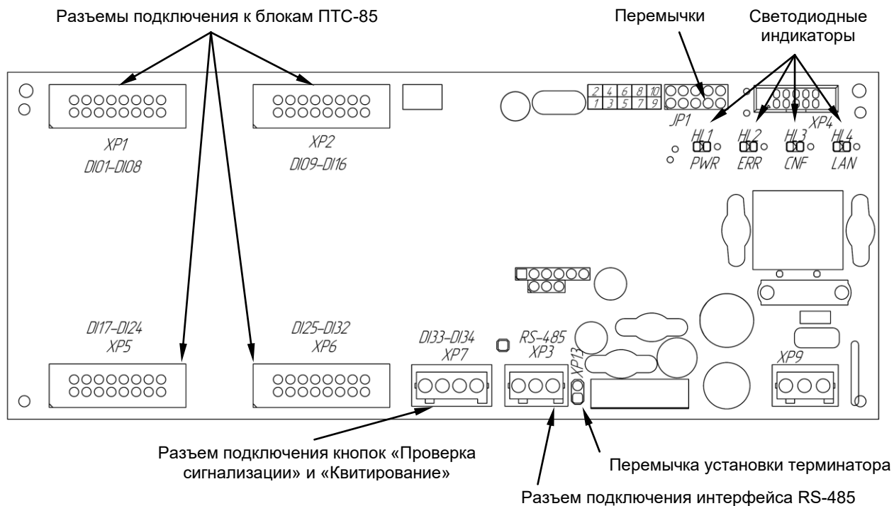
Рисунок. 3.1.3 - Внешний вид блока интерфейса ПТС-32МІ
