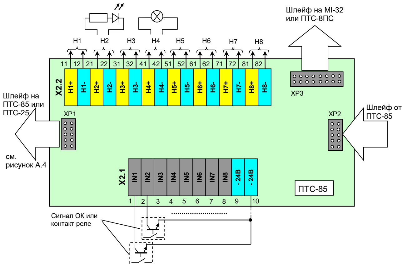
Рисунок. А.2 - Схема внешних соединений и сигналы блока технологической сигнализации ПТС-85
