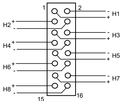
Рисунок. А.3 - Назначение контактов выходного разъема ХР3 блока ПТС-85
