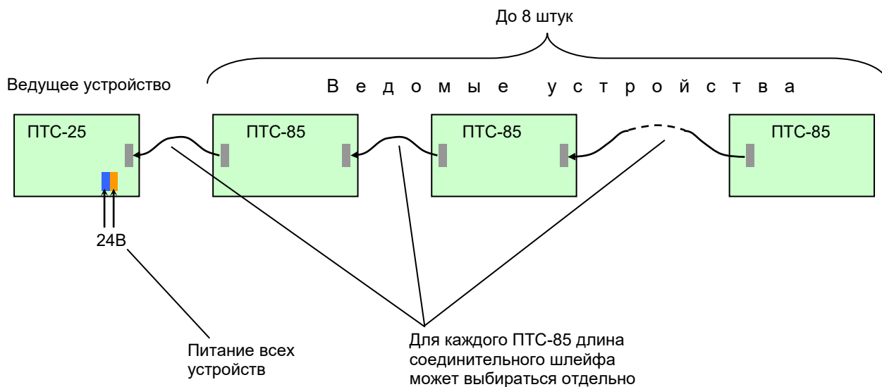
Рисунок. А.4 – Подключение блоков ПТС-85 к ведущему ПТС25
