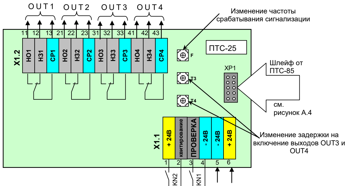
Рисунок. А.1 - Схема внешних соединений и сигналы блока технологической сигнализации ПТС-25
