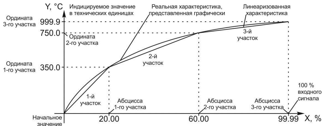
Рисунок 3.2 – График линейризованного сигнала
