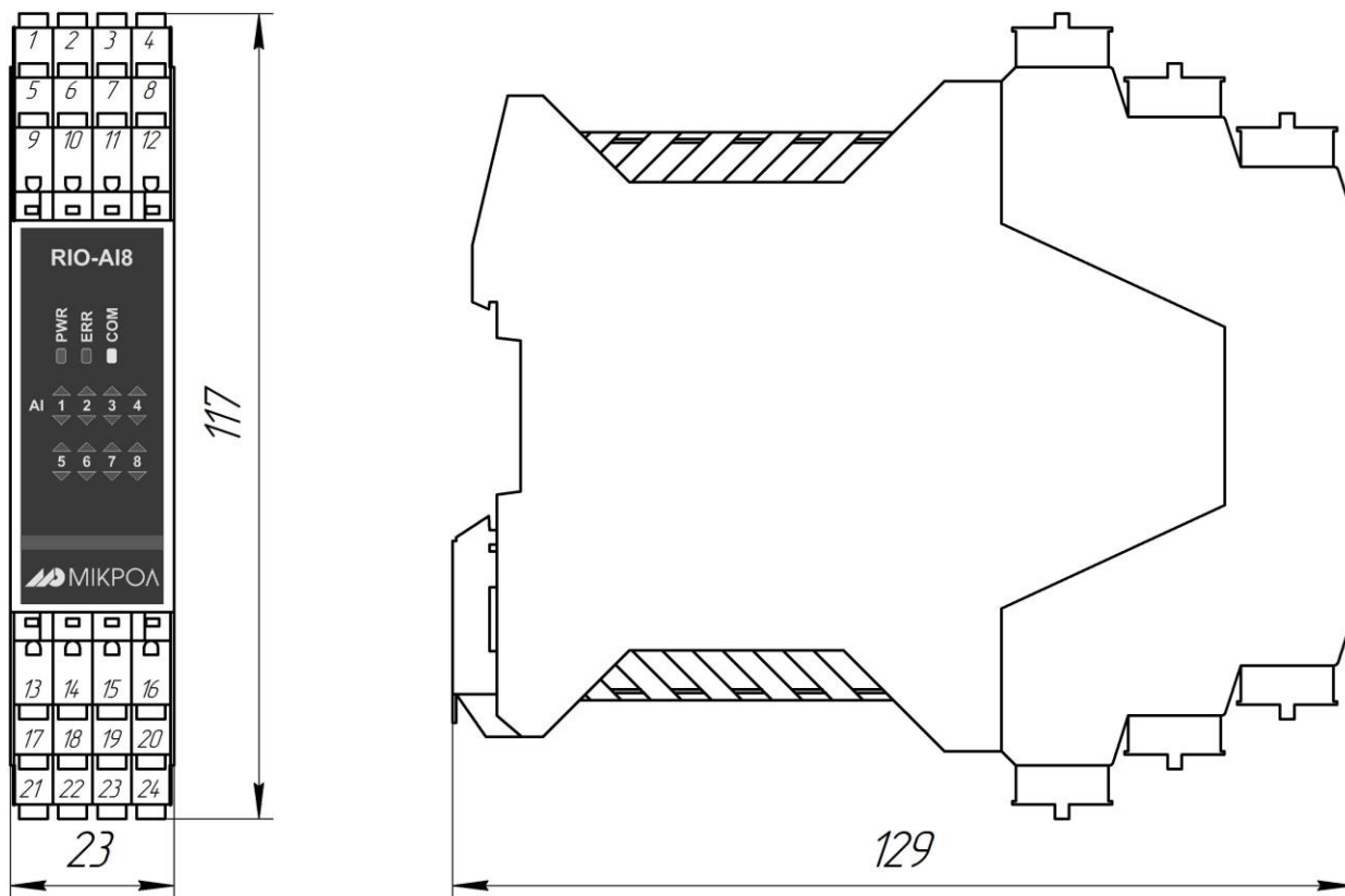
Рисунок А.1 - Габаритные размеры модуля RIO-AIU8
