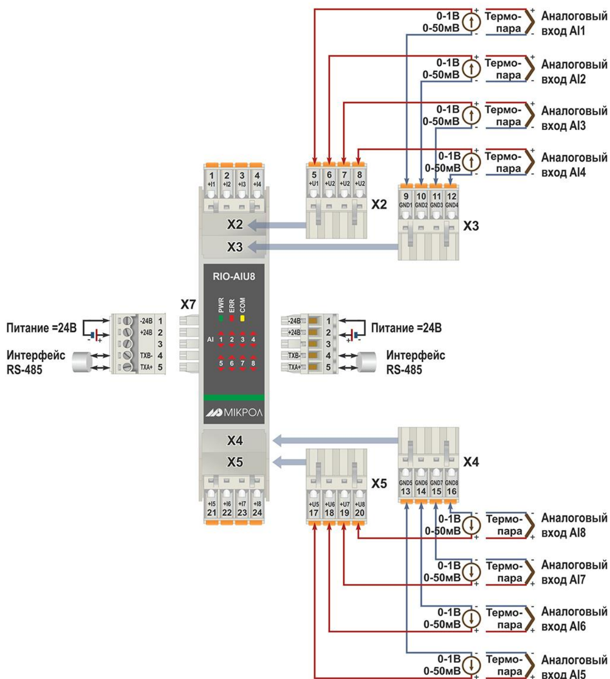
Рисунок Б.2 – Схема внешних соединений для подключения термопар к модулю RIO-AIU8
