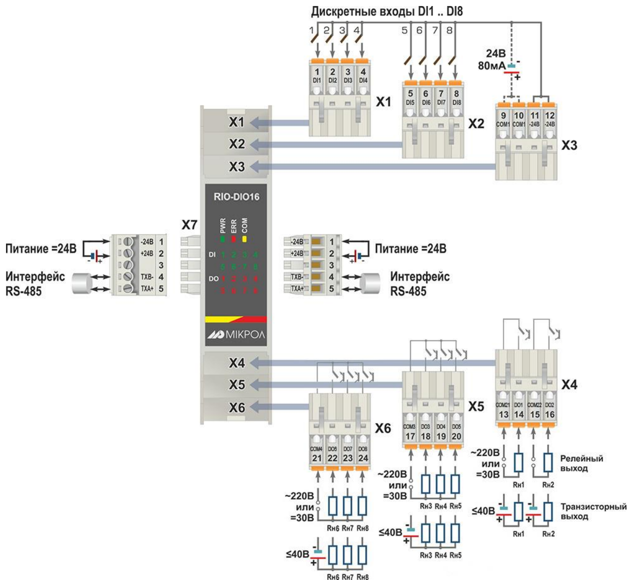
Рисунок Б.1 – Нумерация клемм и сигналы модуля дискретного ввода/вывода RIO-DIO16: а) с внешним источником питания для дискретных входов; б) с внутренним источником питания для дискретных входов
