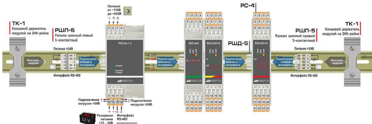
Рисунок Б.2 - Схема внешних соединений RIO-DIO16 с блоком питания и другими модулями
