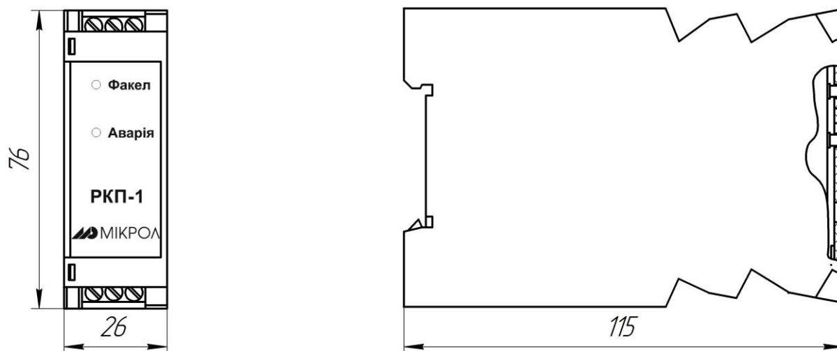
Рисунок 1.1 – Внешний вид и габаритные размеры РКП-1
