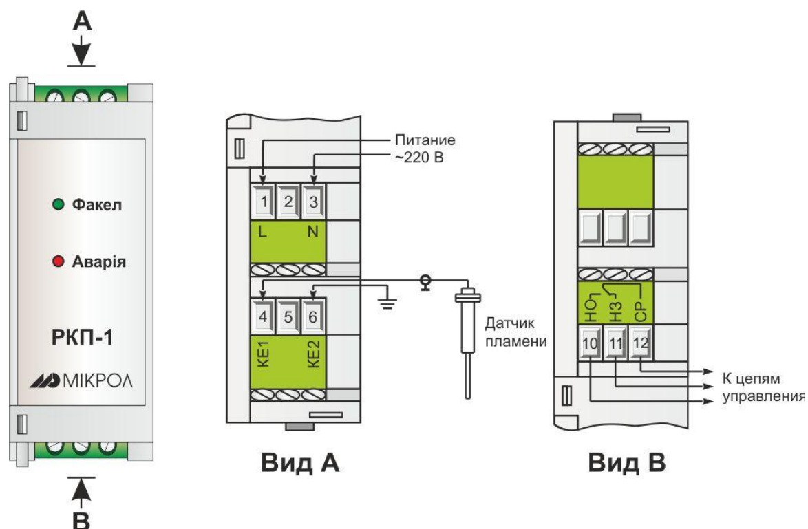
Рисунок 3.2 – Схема внешних соединений РКП-1
