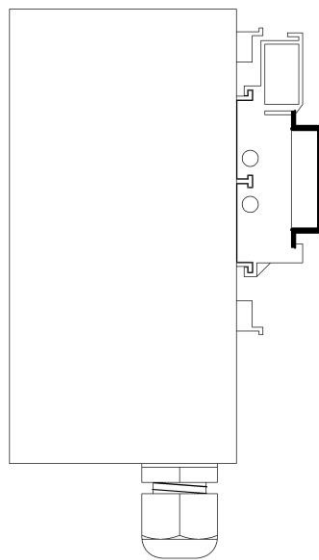
Рисунок 4.1 – Схема установки и снятия блока РСУ-31
