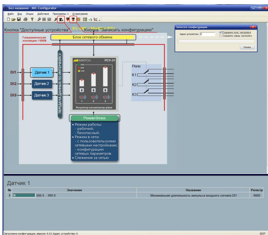
Рисунок 4.5 – Редактирование конфигурации
