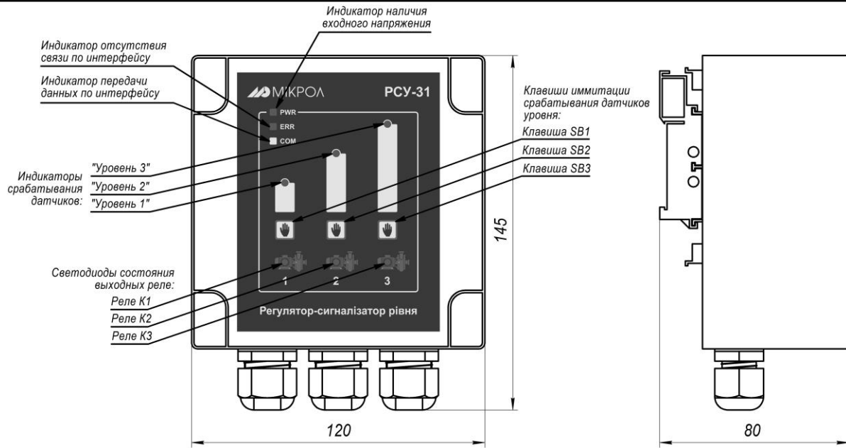
Рисунок 1.4 – Внешний вид и габаритные размеры PCY-31
