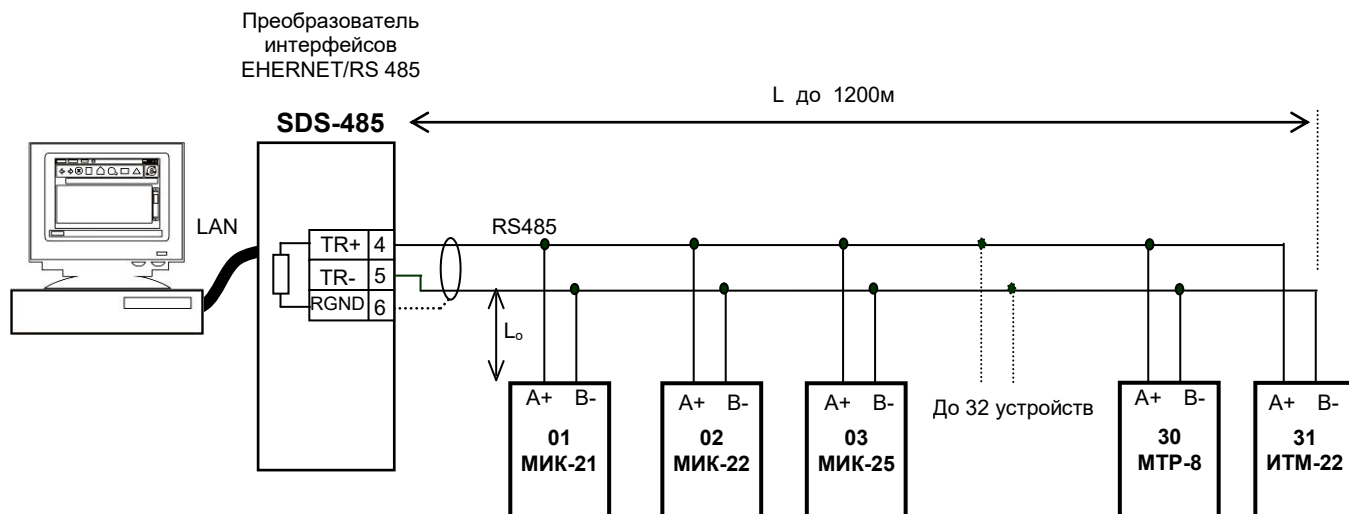
Рисунок В.1 - Организация интерфейсной связи между компьютером и абонентами (устройствами) сети RS-485
