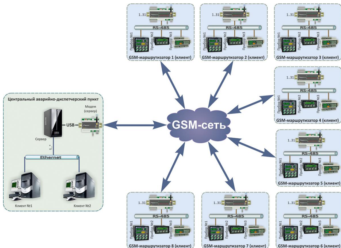
Рисунок 3.3 – Схема системы с Squid-1Н в качестве сервера и восемью удалёнными GSM-маршрутизаторами Squid-2Н
