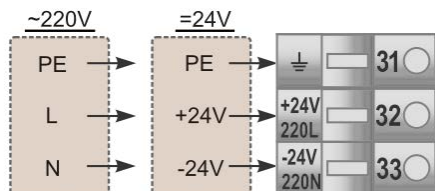
Рисунок А.2 – Расположение внешних соединительных устройства SQUID-2H-4AI-DI8
