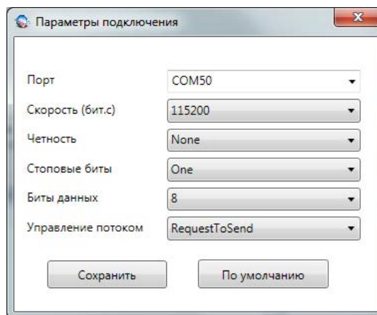
Рисунок 8.26 - Запись настроек в GSM-маршрутизатор Squid-2H
