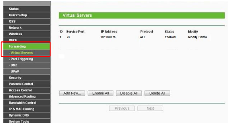
Рисунок 8.13 – Роутер TP-link
