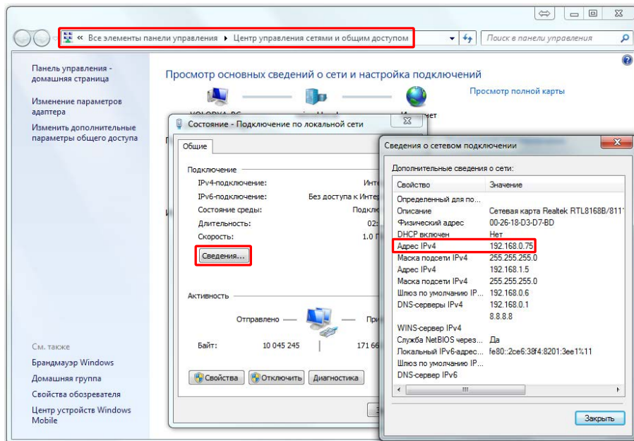
Рисунок 8.14 – Внутренняя IP-адреса
