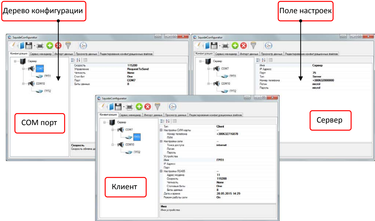
Рисунок 7.4 - Вкладка «Конфигурация»
