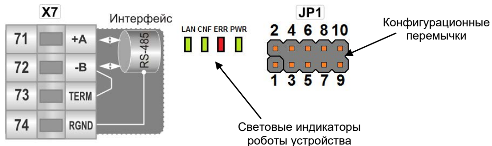
Рисунок А.6 - Подключение интерфейса RS-485 (только УАС-16МІ)
