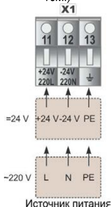
Рисунок А.2 - Подключение к устройству аварийной сигнализации YAC-16 (YAC-16MI) питания 220 В или 24 В
