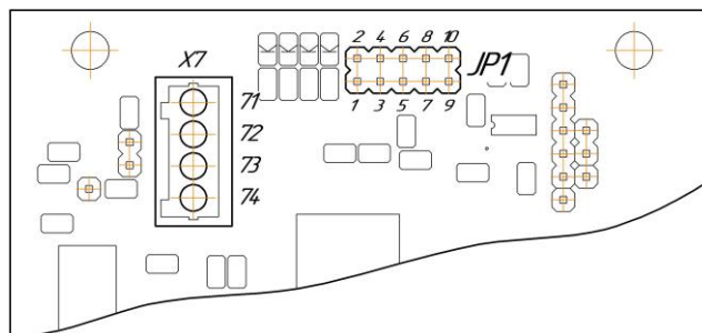
Рисунок А.7 – Плата модуля интерфейса МІ (только УАС-16МІ)
