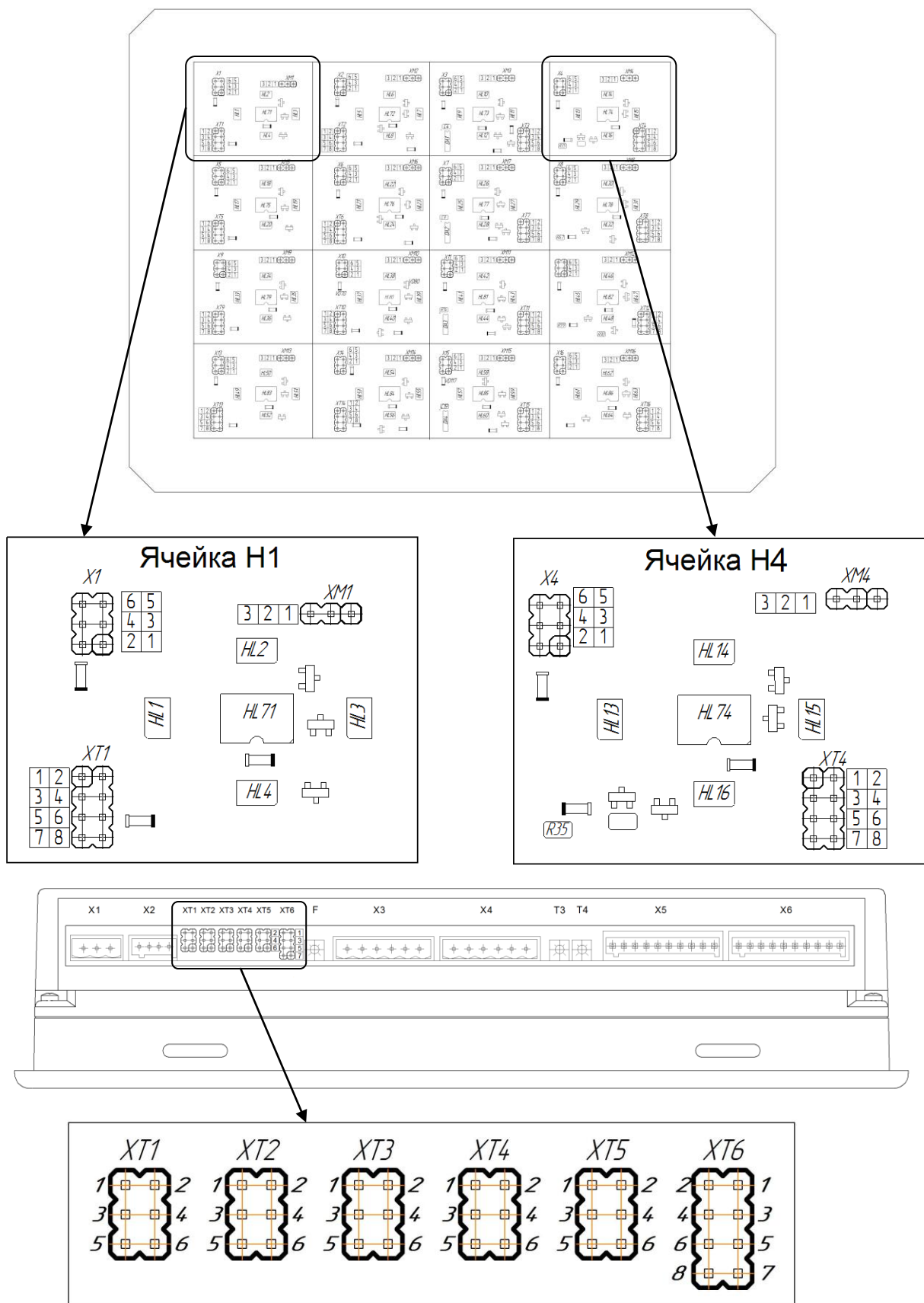
Рисунок 2.2 – Расположение перемычек на плате устройства УАС-16(УАС-16М)
