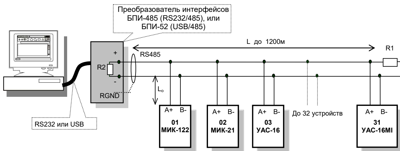
Рисунок Б.1.1 - Организация интерфейсной связи между компьютером и регуляторами
