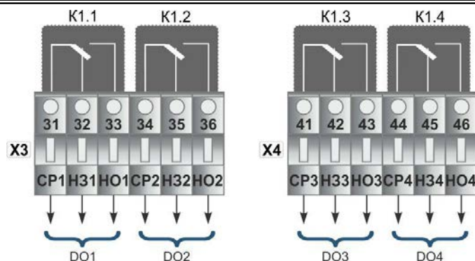
Рисунок А.4 - Подключение дискретных выходов устройства УАС-16 (УАС-16МІ) (внешняя световая или звуковая сигнализация, а также сигнал каскадирования)
