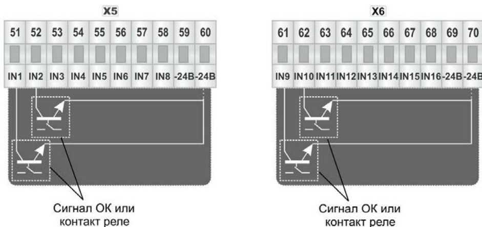
Рисунок А.5 - Подключение дискретных входов устройства УАС-16(УАС-16МІ) (от двухпозиционных датчиков)
