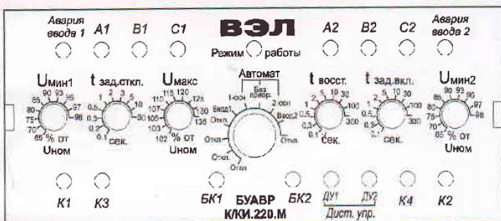
Рис. 3 Расположение органов управления и индикации БУАВР.К и БУАВР.КИ
