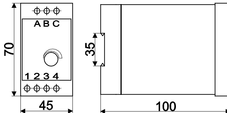
Рисунок 1 - Габаритные и установочные размеры реле
