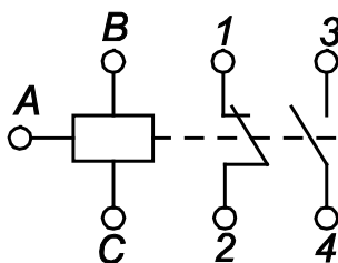
Рисунок 2 – Схема подключения реле
