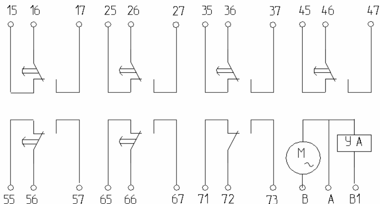
Рисунок 3 – Схема электрическая принципиальная реле ВС43-3
