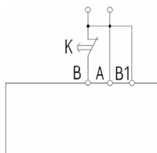
Рисунок 4 – Схема электрическая принципиальная реле ВС43-3
