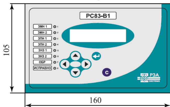
Вид спереди
