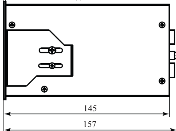
Вид слева
