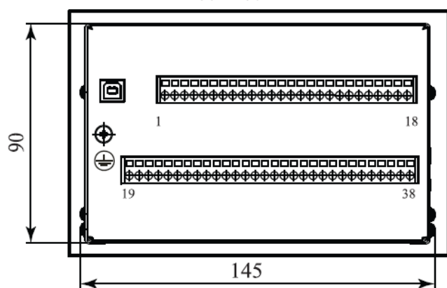
Вид сзади
