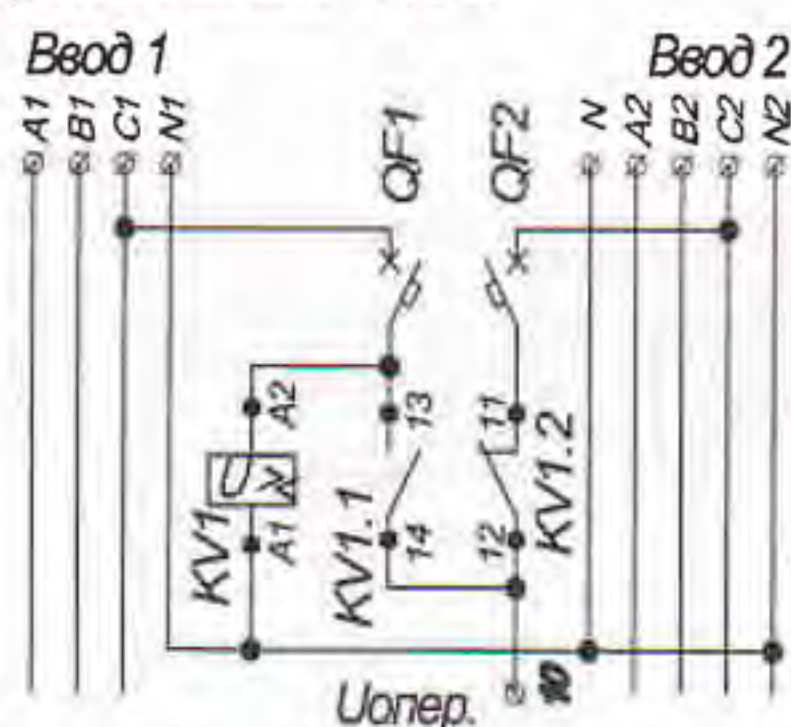
Рис. 6 Схема получения оперативного питания с использованием реле напряжения и UPS
