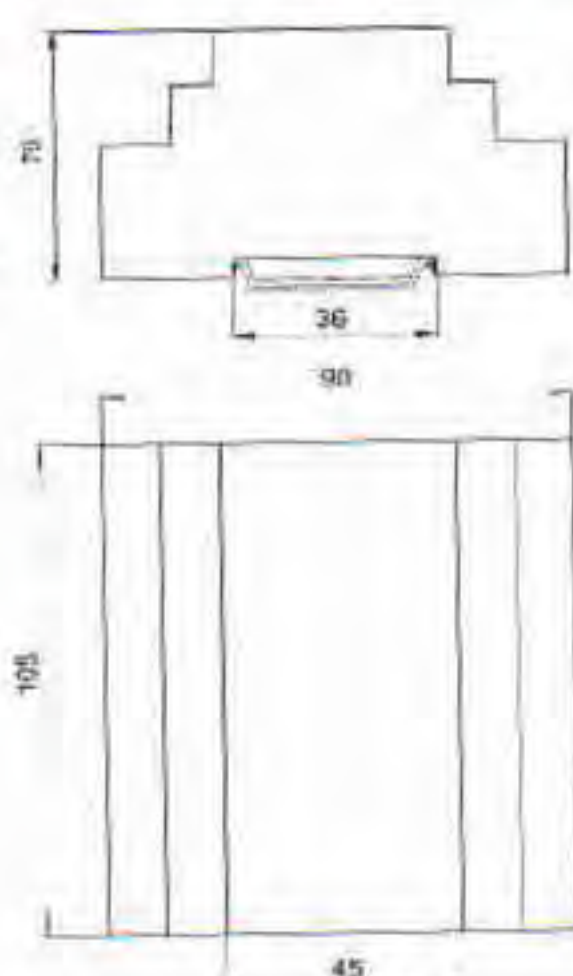
Рис.2 Габаритные и установочные размеры БУАВР
