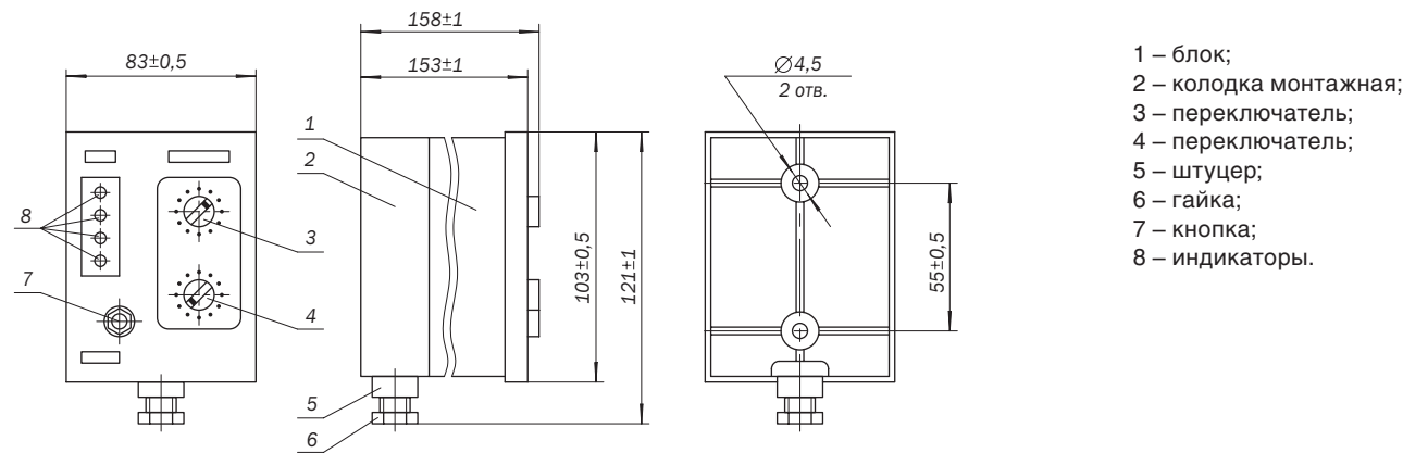
Рис.1. Блок управления типа БИВ-11
