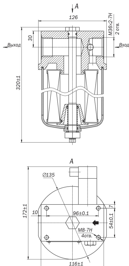
Рис.1. Фильтр сливной типа ЗФС
