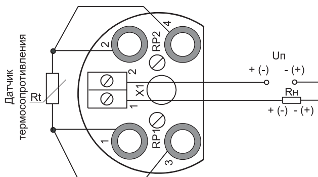
Схема подключения преобразователя PSA-02.02.XX.XX.XX
