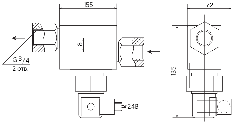
Рис.1. Сигнализатор стружки
