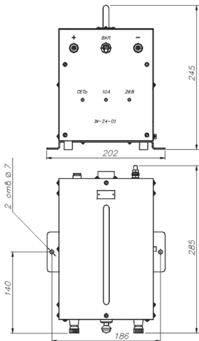
Рисунок 4 - Габаритно-установочные размеры
