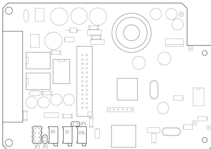
Рисунок 5.2 - Расположение перемычек настройки и органов регулировки выходного сигнала на плате процессора БРУ-7 (БРУ-7К1) внутри блока
