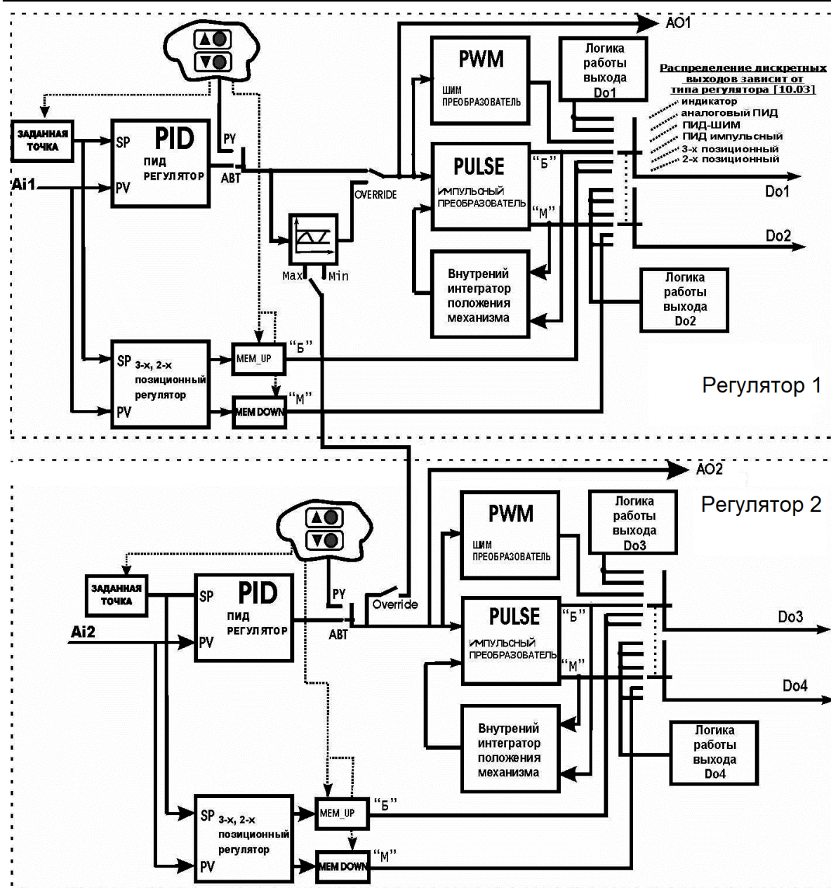
Рисунок 3.3 - Функциональная схема блока регулирования
