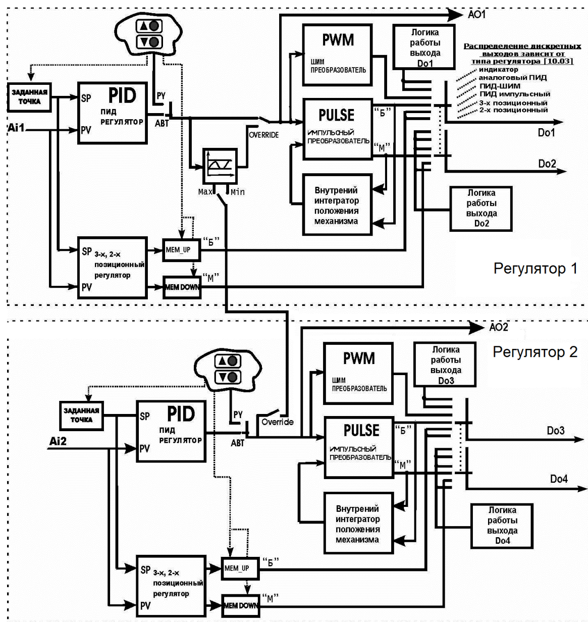
Рисунок 3.3 - Функциональная схема блока регулирования
