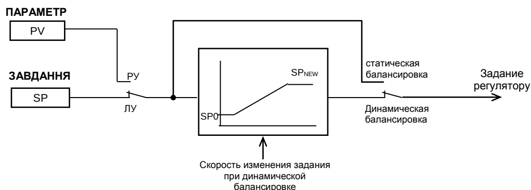
Рисунок 4.2 – Функциональная схема балансировок регулятора МИК-122Н
