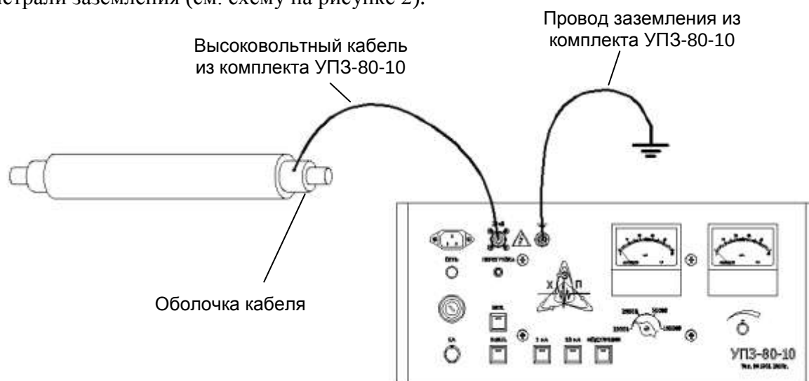
Рисунок 2. Схема подключения УПЗ-80-10 для испытания оболочки и точной локализации места повреждения.
