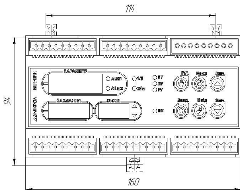
Вид спереди
