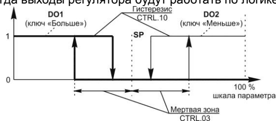
Рисунок 3.17 - График работы дискретных выходов 3-х позиционного регулятора с использованием зоны нечувствительности (CTRL.03)
