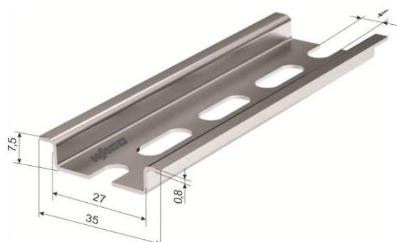
Рисунок А.3 – Внешний вид и размеры DIN-рейки Wago
