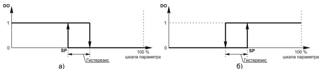
Рисунок 3.16 – Пример работы выходного устройства: а) по логике обратного 2-х позиционного управления п. CTRL.00=0000, п. CTRL.01=0000, б) по логике прямого 2-х позиционного управления п. CTRL.00=0000, п. CTRL.01=0001
