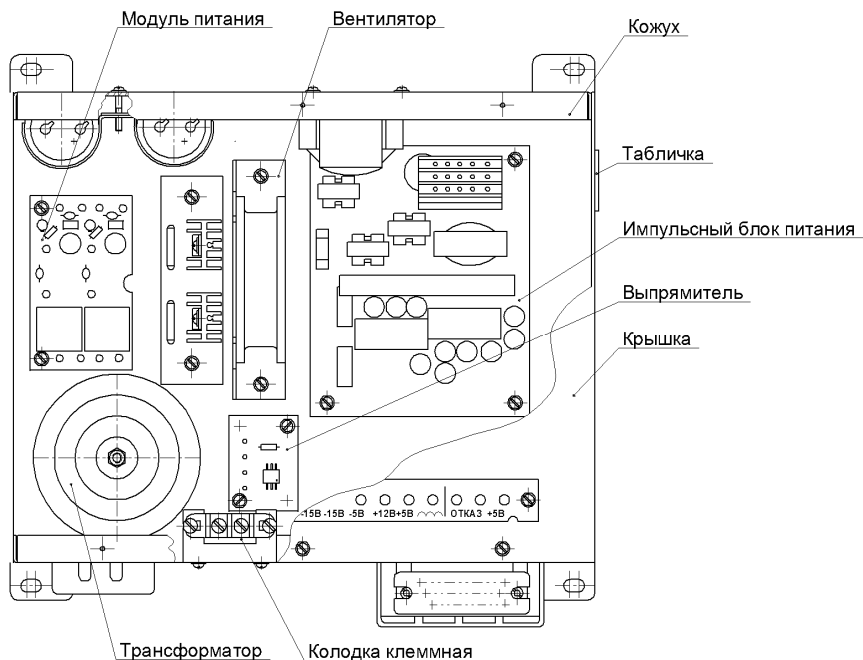
Рисунок 2 – Блок питания стабилизирующий БПС-7. Вид внутри.
