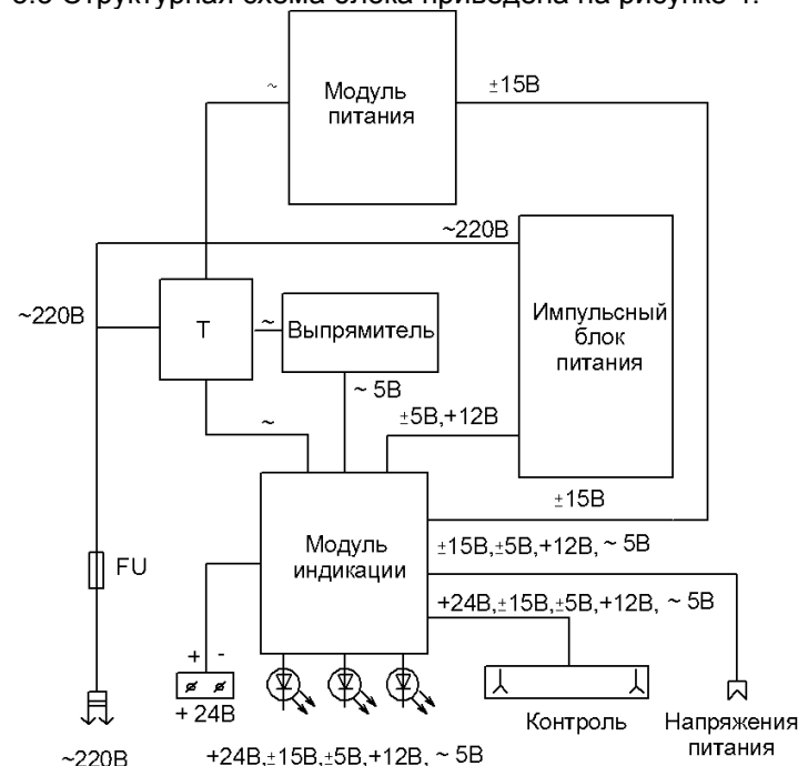
Рисунок 4 – Блок питания стабилизирующий БПС-7. Схема структурная.
