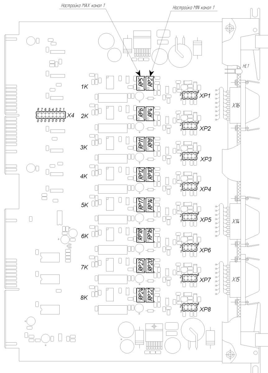
Рисунок 2 – Модуль цифро-аналогового преобразования ЦАП8. Внешний вид.
