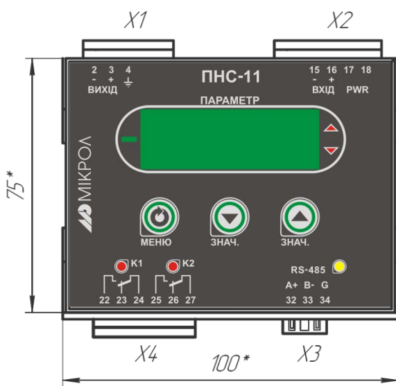
Рисунок А.1 – Внешний вид передней панели преобразователя ПНС-11
