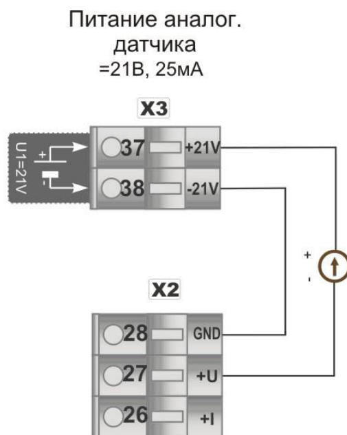
Рисунок Б.2 - Подключение к индикатору ИТМ-111 аналоговых датчиков с пассивными выходами
