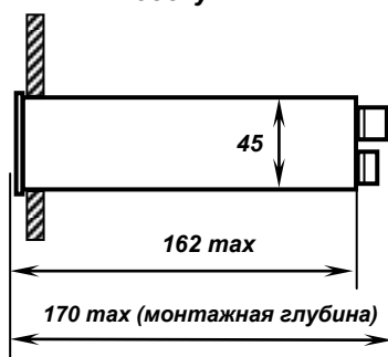
Рисунок А.2 - Габаритные размеры
