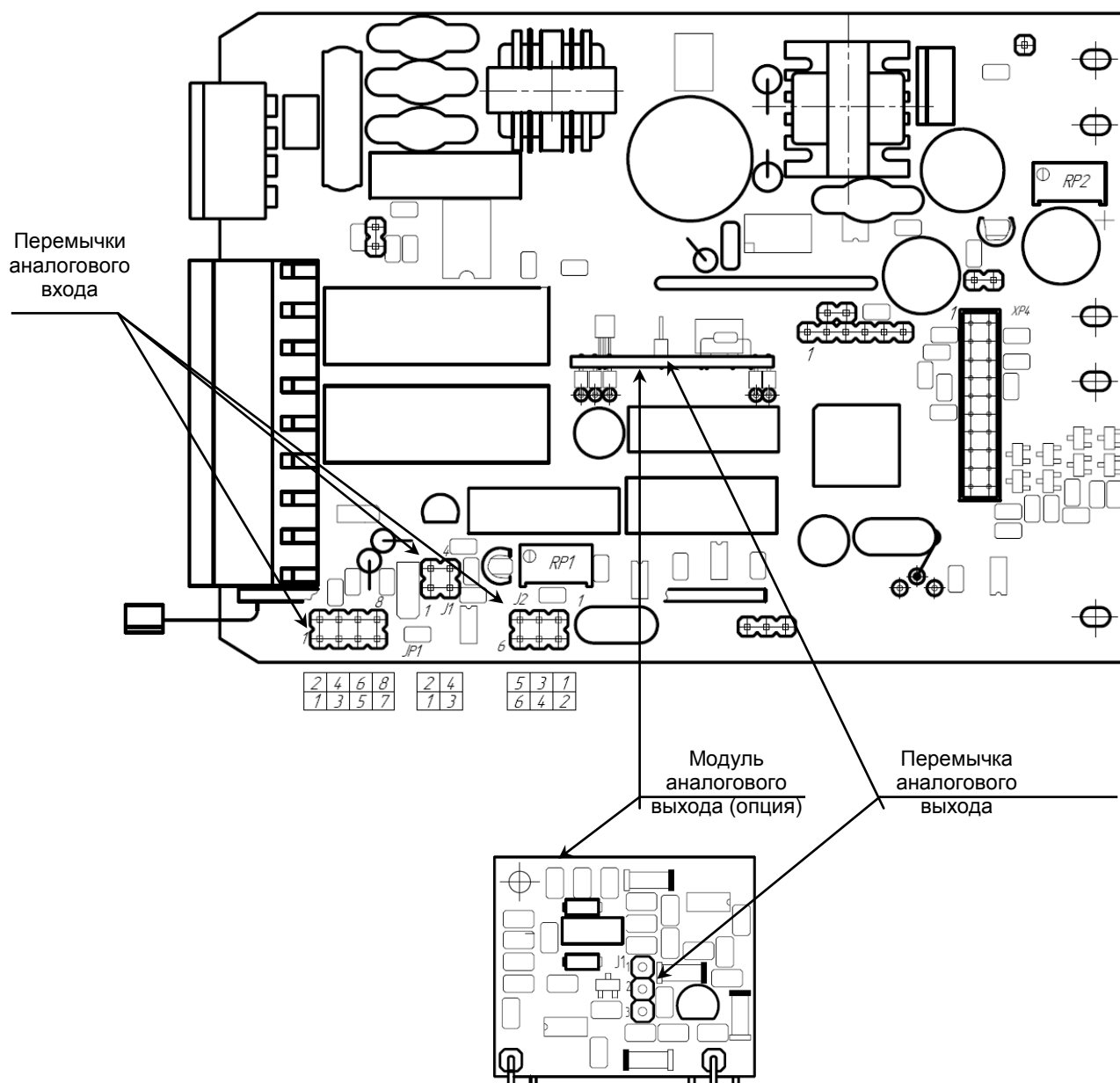
Рисунок 4.4 – Положение перемычек на плате процессора и на модуле аналогового выхода
