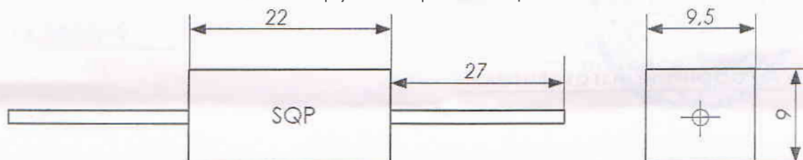
Рис.3 Наружный резистор
