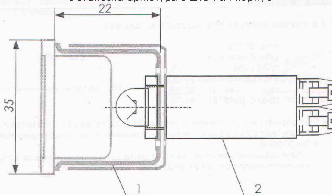
Рис.4 Установка арматуры в штатный корпус
