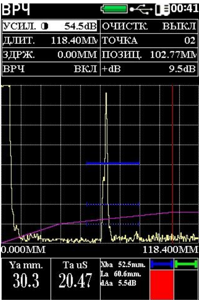
Режим настройки и работы с использованием ВРЧ.
