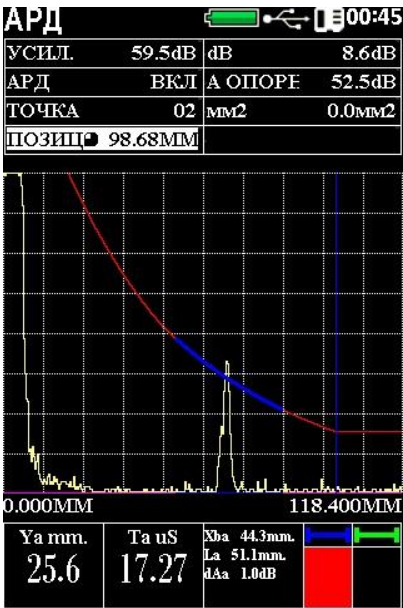
Режим настройки и работы с использованием АРД-диаграмм в вертикальной (портретной) ориентации.
