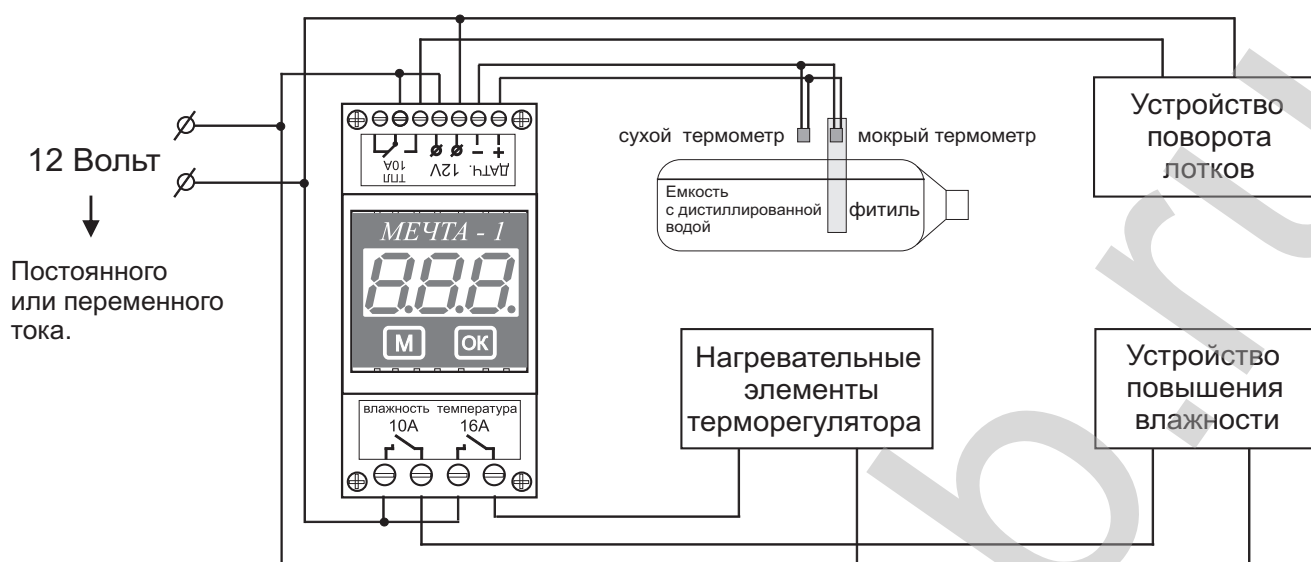
Рис.1 Монтажная схема с не реверсивным двигателем устройства поворота лотков (с кулачковым механизмом и т.д.).
