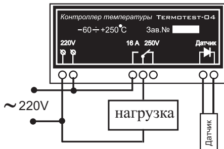
Рис.2 Схема подключения.
