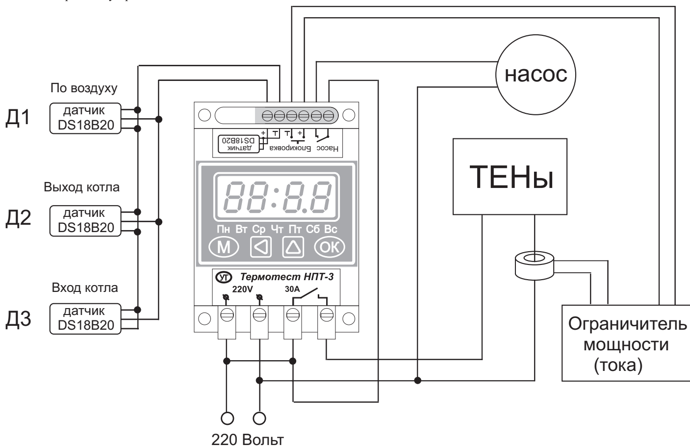
Рис 1. Типовая схема включения терморегулятора. Ограничитель мощности устанавливается по необходимости, если не нужен то исключается из схемы.
