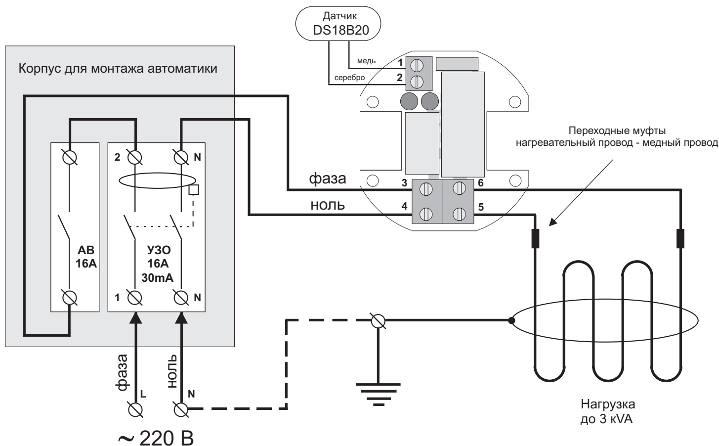
Рисунок 1. Электрическая схема монтажа системы “теплый пол”.
