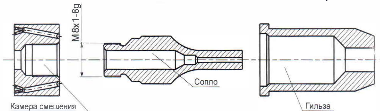
Мундштуки короткие цилиндрические с кольцевой щелью
