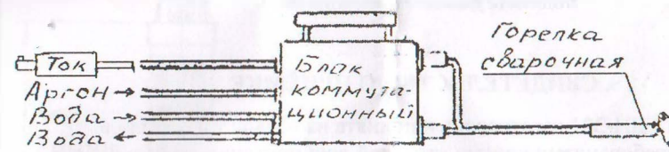
Рис.1 Блок коммутационный
