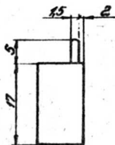
Разметка печатной платы
