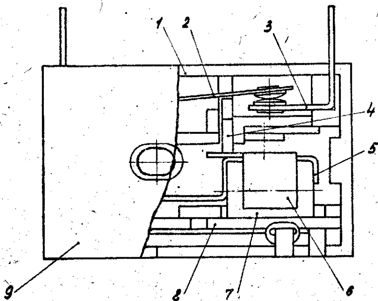
Рис. 4. Устройство реле TPM12-1, TM12-2
