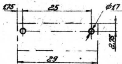
Разметка печатной платы
